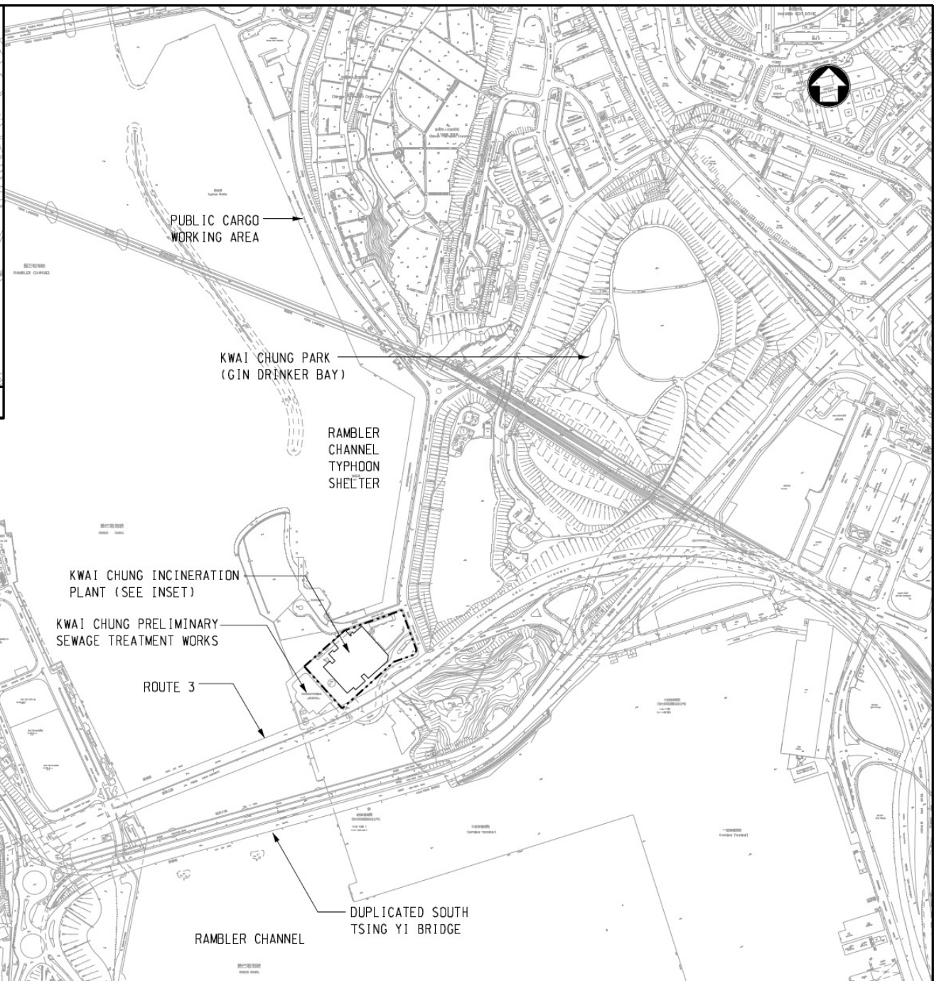
圖1: 葵涌垃圾焚化爐拆卸工程的位置圖及其設計佈局
